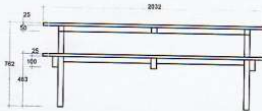
ELEVATION B
