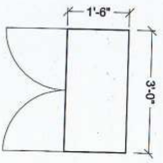
PLAN(07 Nos.)
