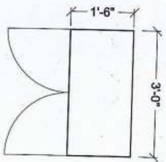
PLAN(07 Nos.)
